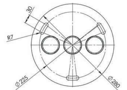
ДТУ178с7 Стэм ДТУ-178-АФ-90Вт-2,7-тройной
