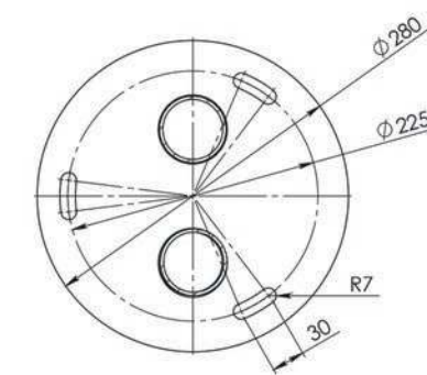
ДТУ178с6 Стэм ДТУ-178-АФ-70Вт-2,7-двойной
