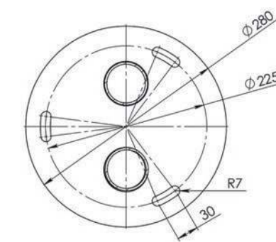
ДТУ178с5 Стэм ДТУ-178-АФ-50Вт-1,9-двойной
