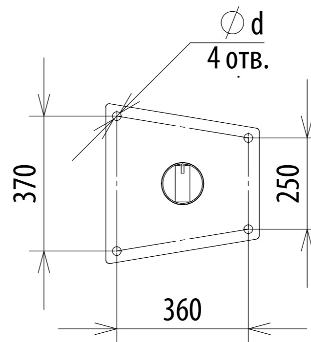
Фланец
