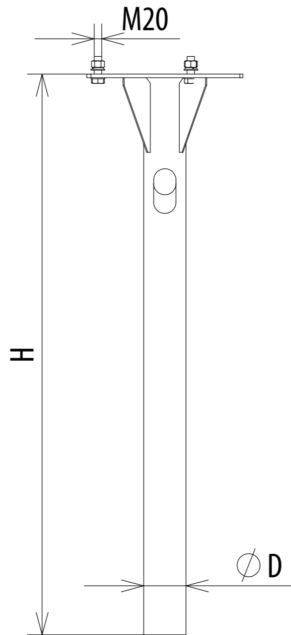
ОПТсФ4-ТРП -Опора подземная трубная с трапецевидным фланцем
