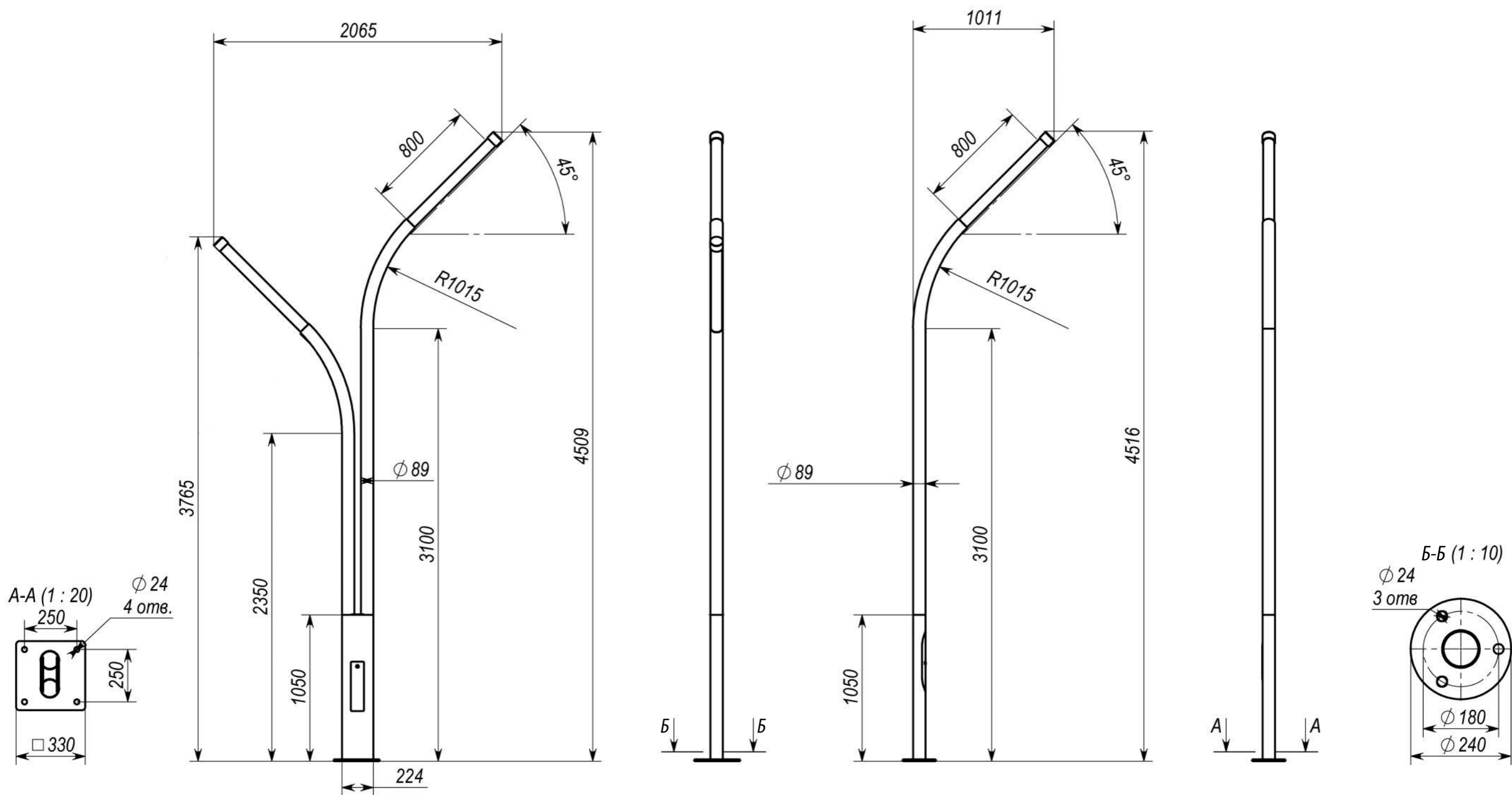
Светодиодный светильник Прибой ДТУ-68-АФ
