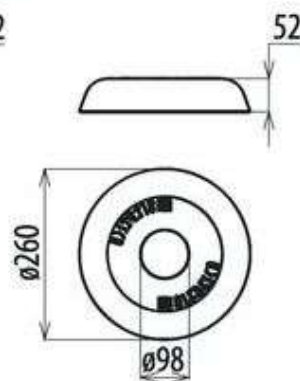
КРШ-d260-3Y
