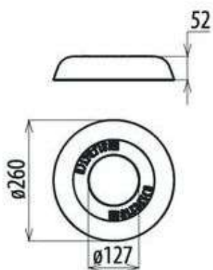
КРШ-d260-1Y
