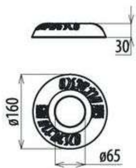
КРШ-d160-1Y
