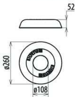
КРШ-d260-2Y
