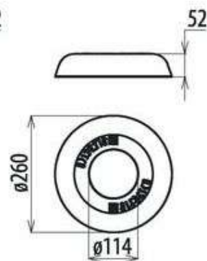
КРШ-d260-4Y
