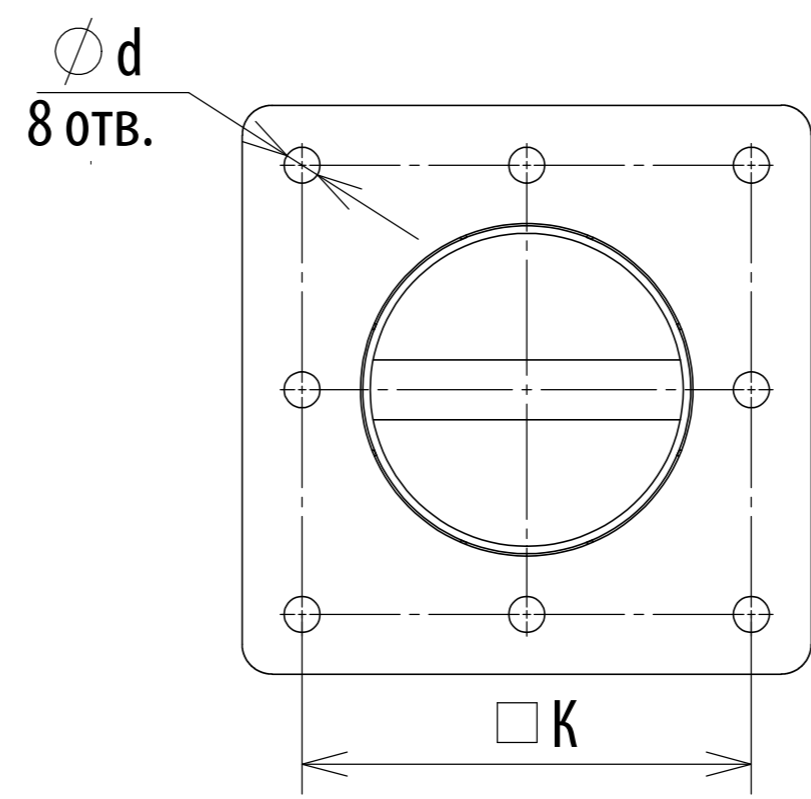
Фланец
